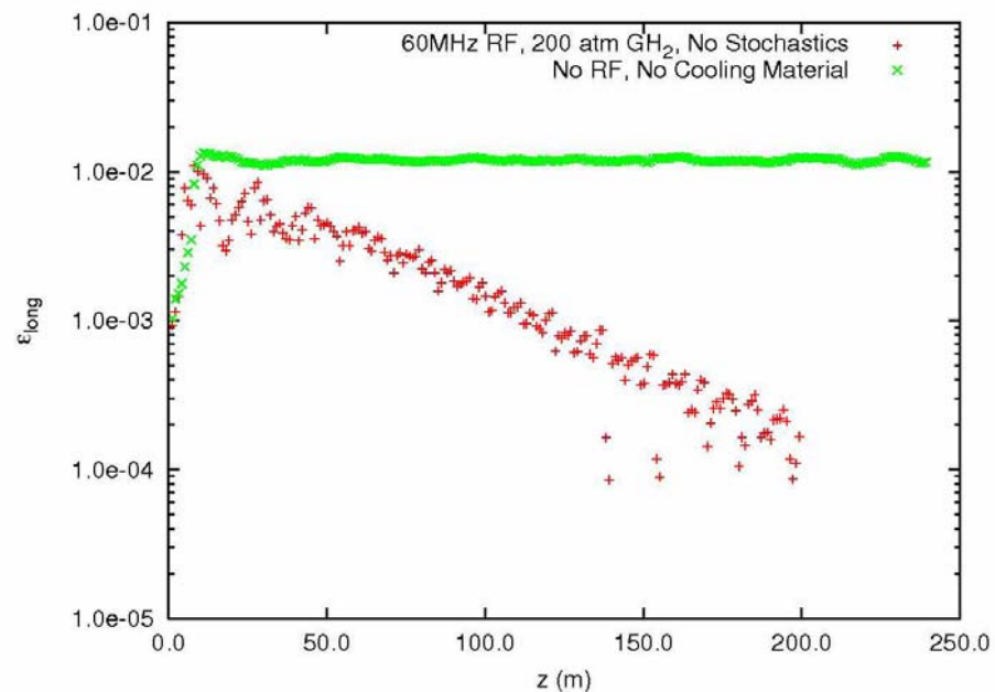
Longitudinal emittance
