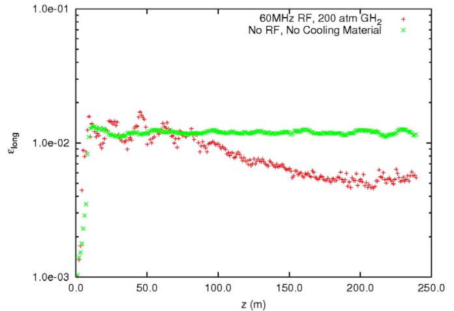
Longitudinal emittance
